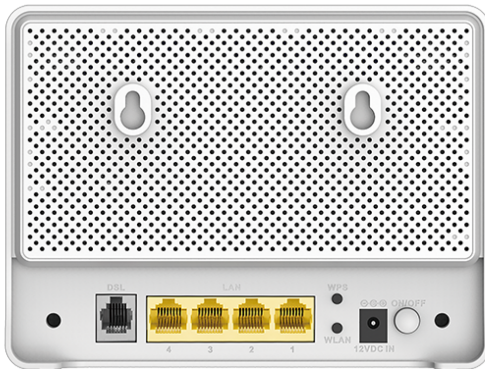
Рисунок 3. Вид задней панели DSL-224.
