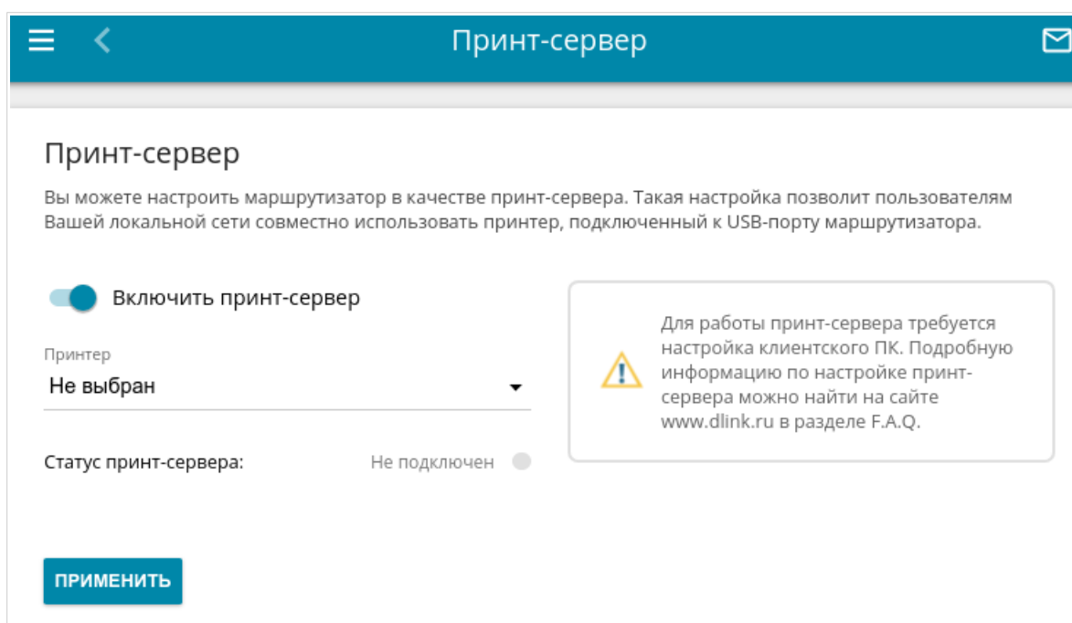
Рисунок 153. Страница Принт-сервер .
