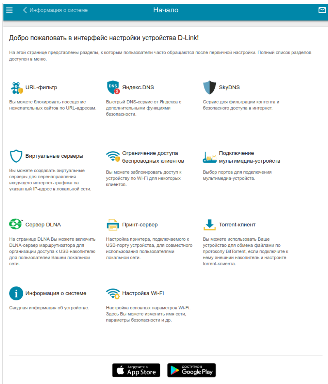
Рисунок 26. Страница Начало .
