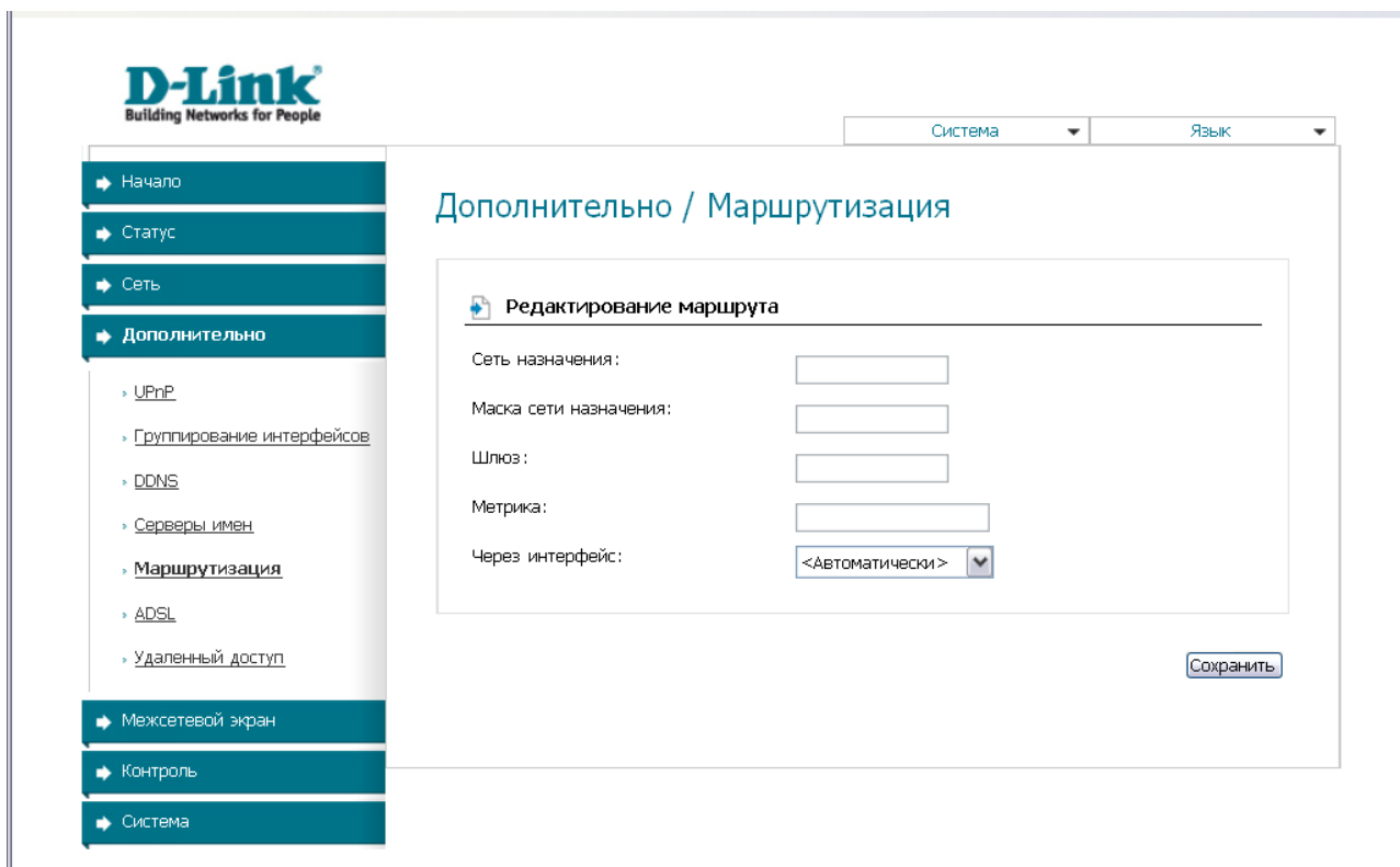
Рисунок 33. Страница добавления статического маршрута.
