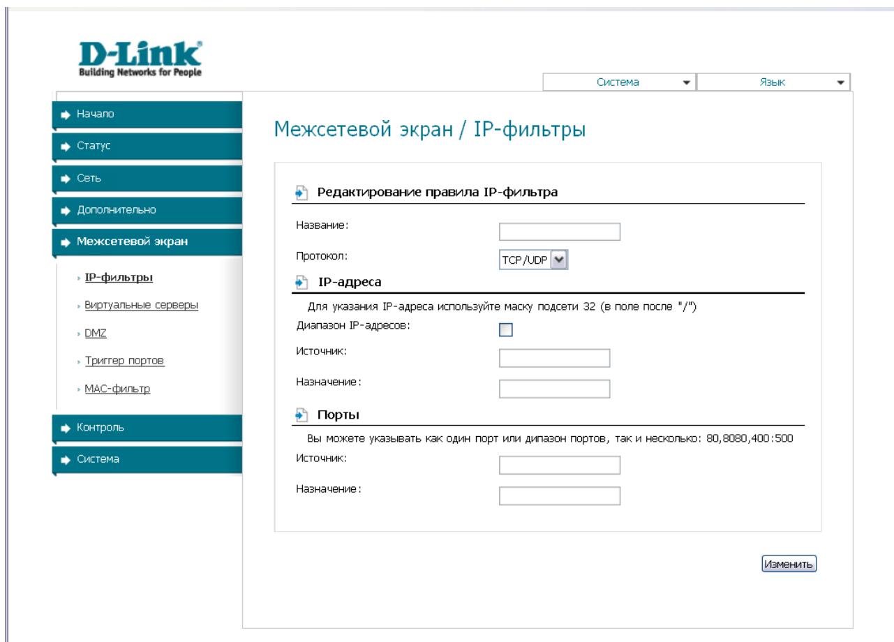
Рисунок 38. Страница добавления правила для обработки сетевых пакетов.
