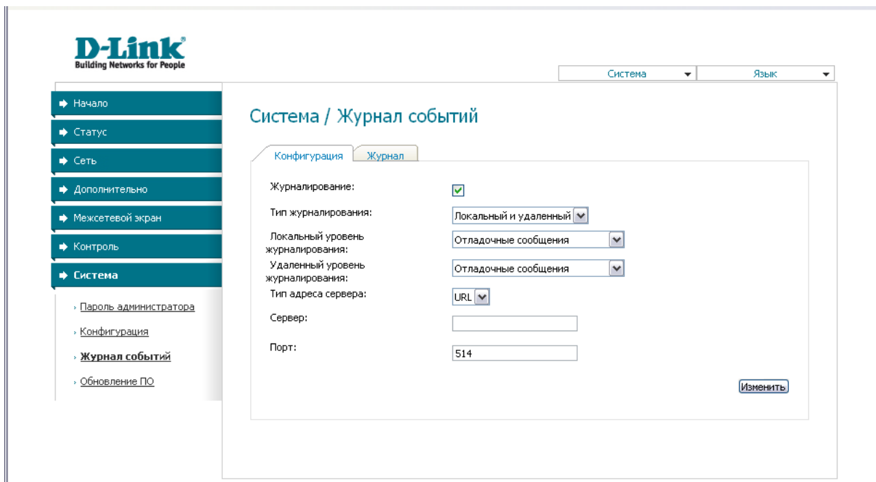
Рисунок 52. Страница Система / Журнал событий. Закладка Конфигурация.
