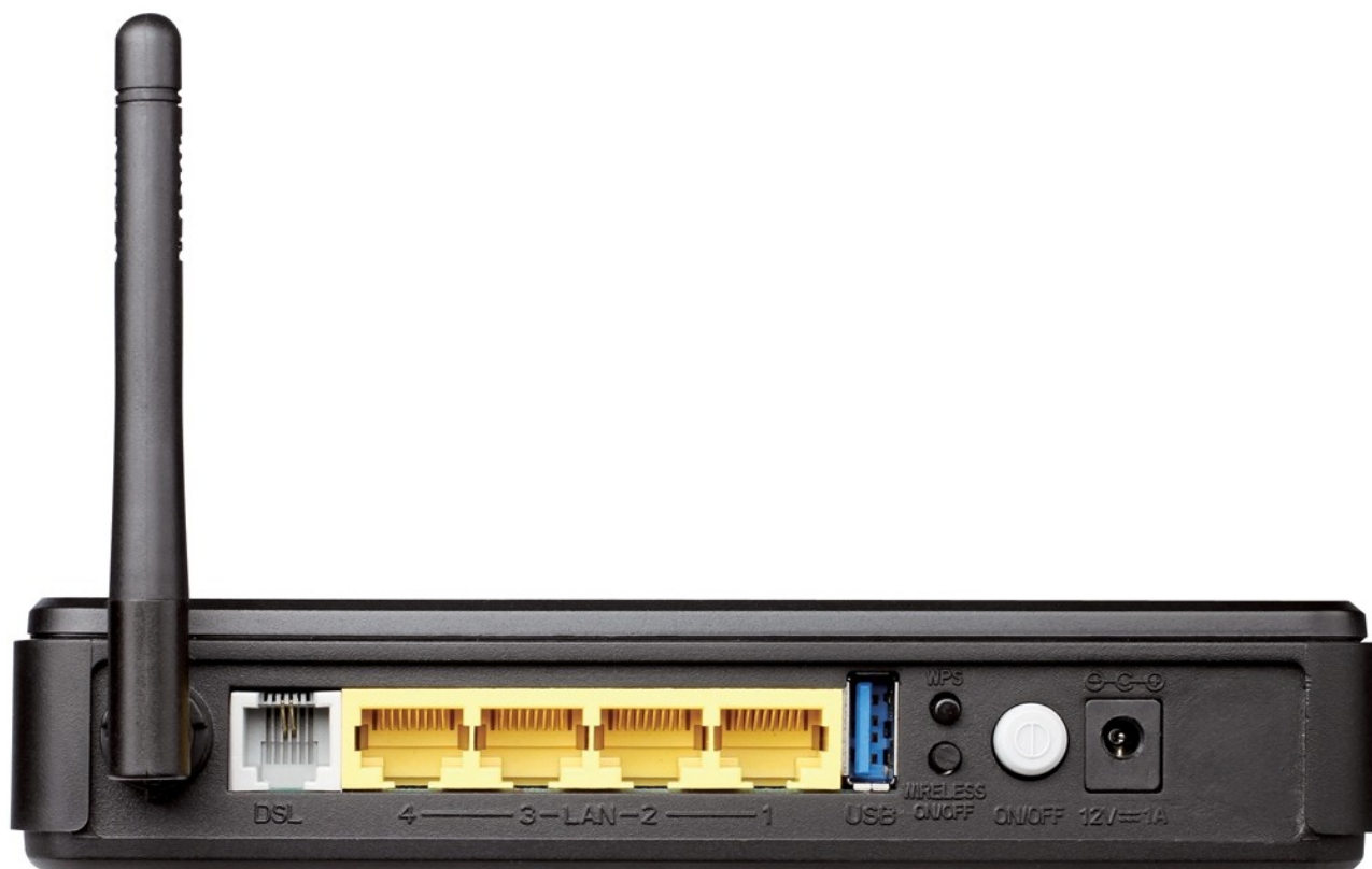
Рисунок 2. Вид задней панели DSL-2650U.
