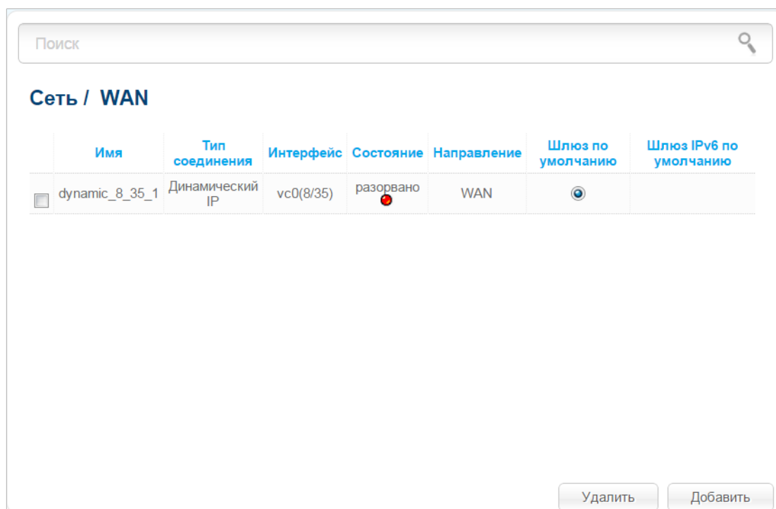
Рисунок 49. Страница Сеть / WAN .
