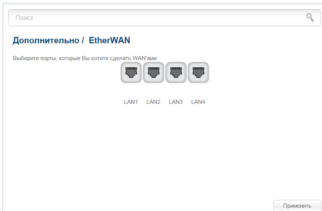
Рисунок 77. Страница Дополнительно / EtherWAN .
