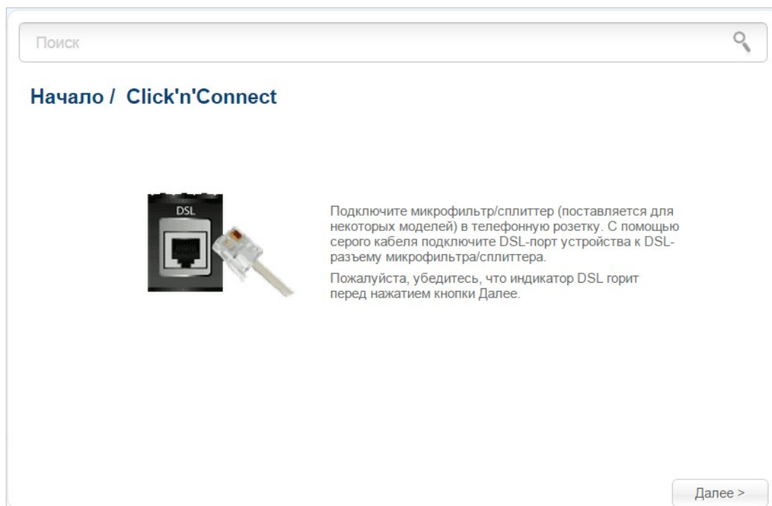
Рисунок 24. Настройка WAN-соединения.
