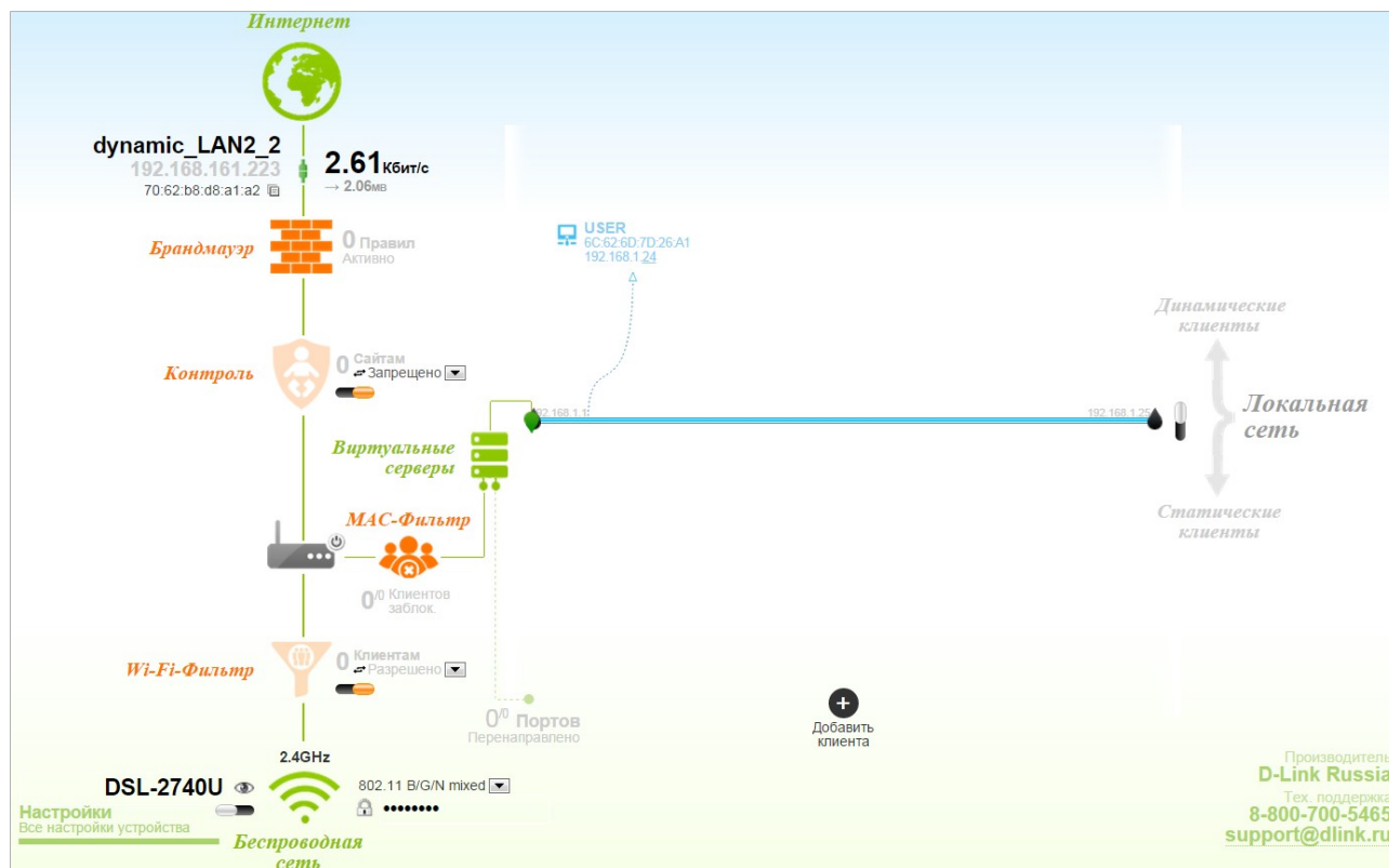
Рисунок 23. Страница Мониторинг .
