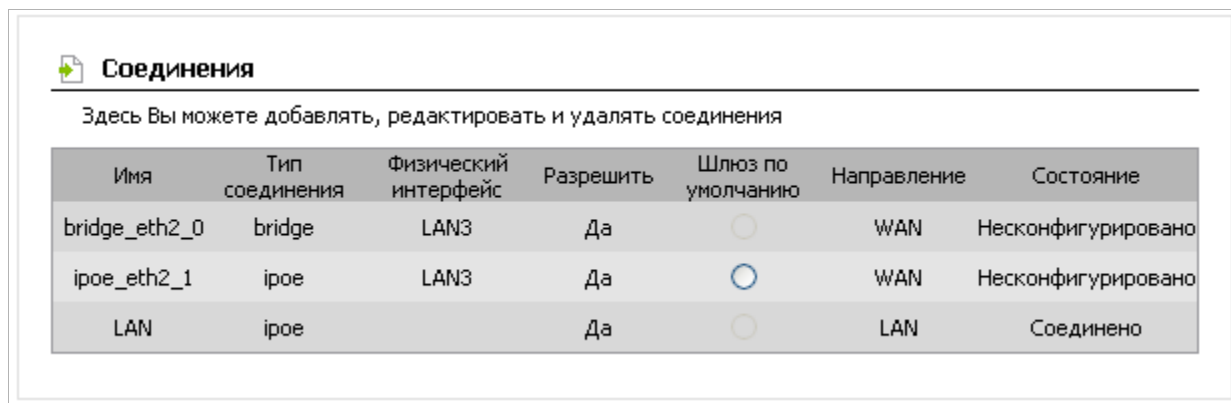
Рисунок 85. Два WAN-соединения для одного физического интерфейса.
