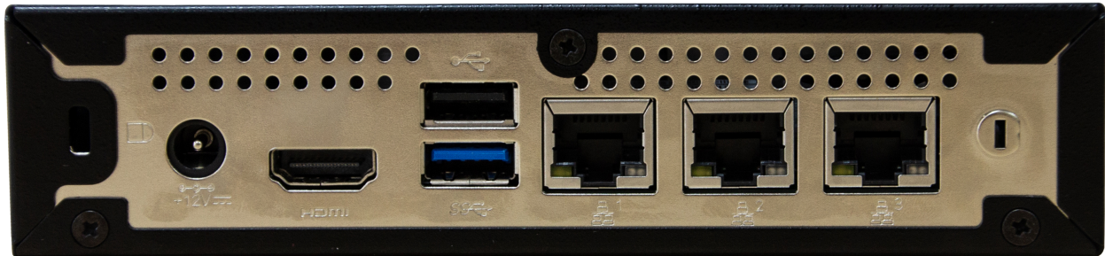
Рисунок 1. Вид задней панели.
