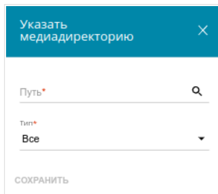
Рисунок 108. Добавление медиадиректории.
