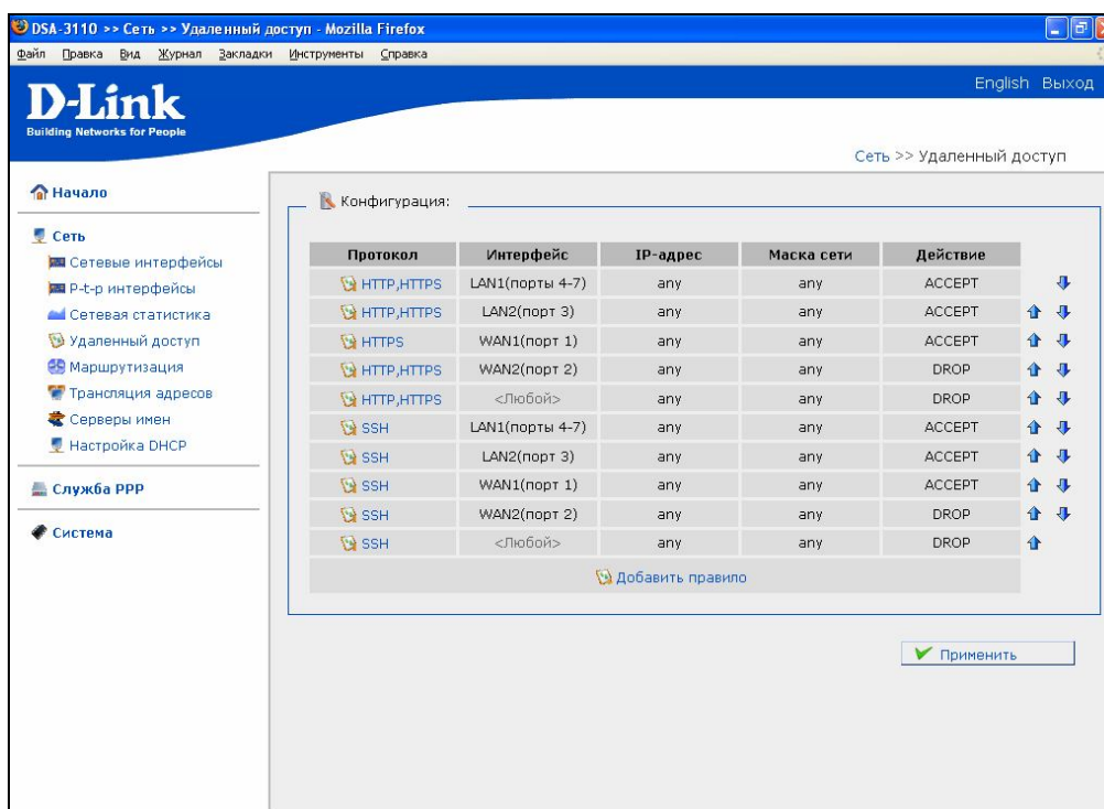
Рисунок 17. Удаленный доступ
