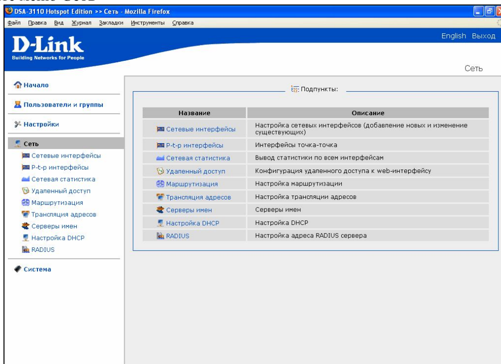
Рисунок 10. Меню Сеть.
