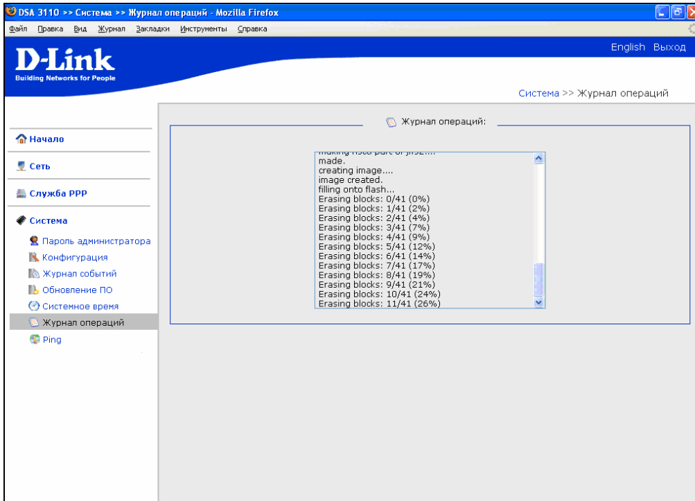
Рисунок 45. Журнал операций
