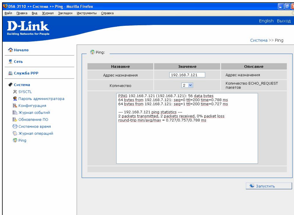
Рисунок 46. Ping (эхо-запрос)
