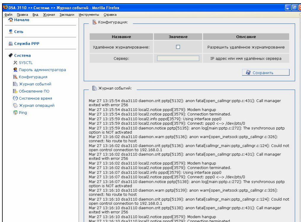
Рисунок 42. Журнал событий
