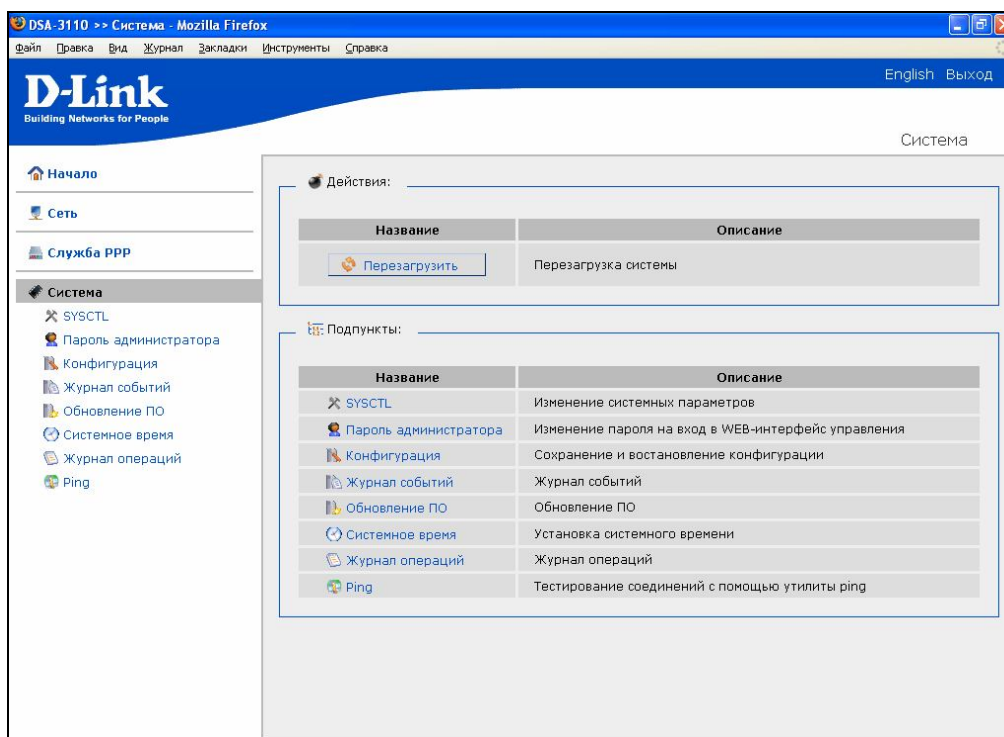
Рисунок 39. Меню Система.
