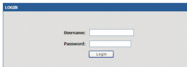
Рис.7 Сообщение аутентификации
