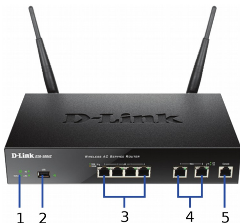
Рис. 1. Передняя панель DSR-500AC
