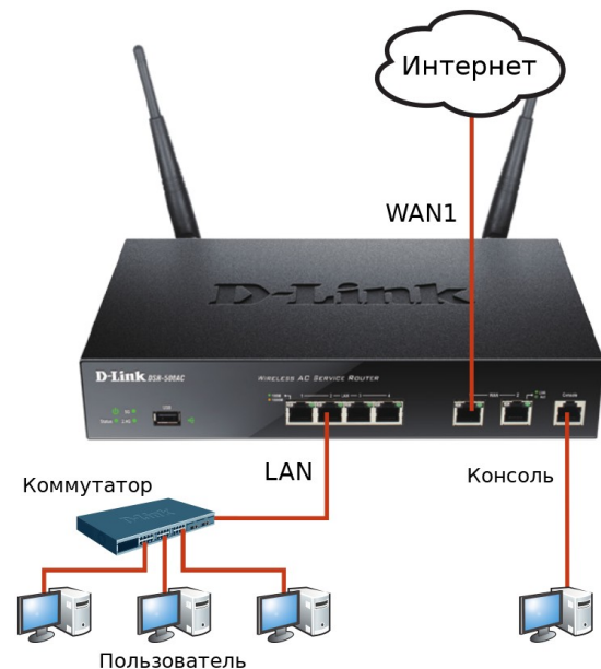
Рис. 5. Пример подключения кабелей
