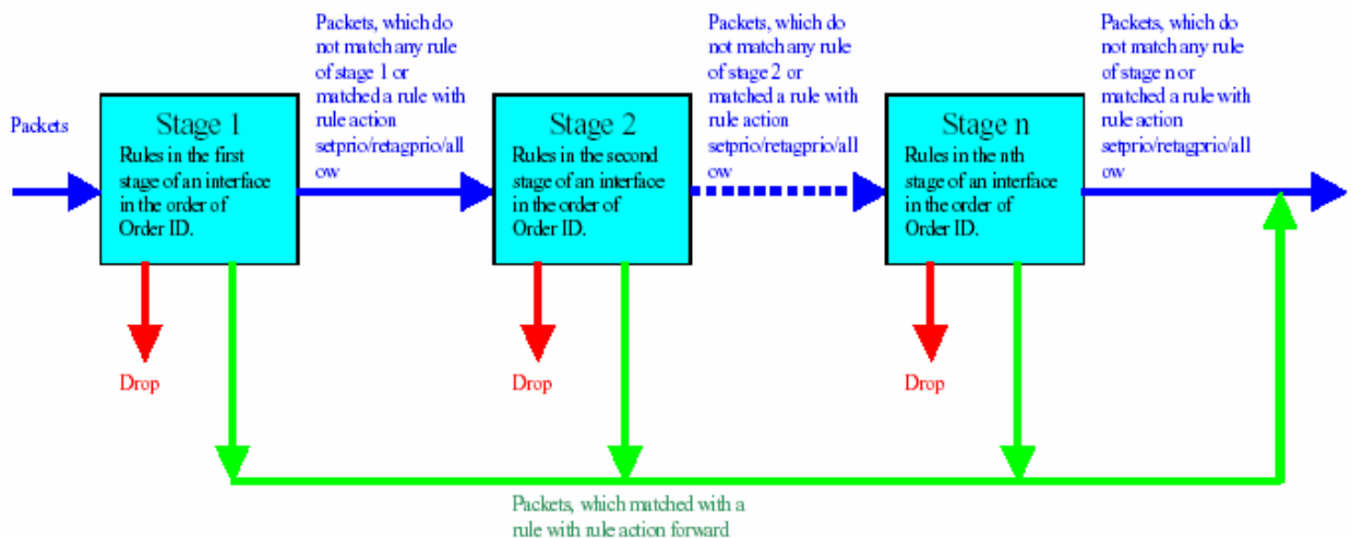
Рисунок 9-4: Многоэтапность обработки пакетов.
