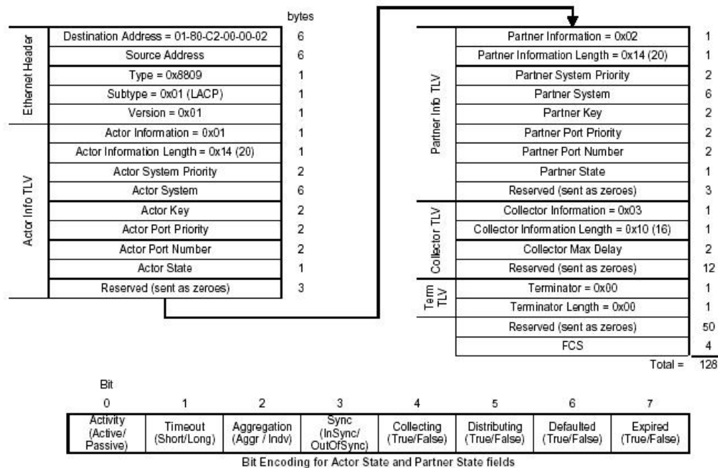
Рисунок 6-7: Формат LACP кадра.
