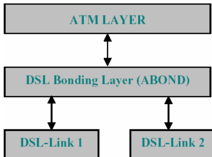
Рисунок 5-1: ATM стек.
