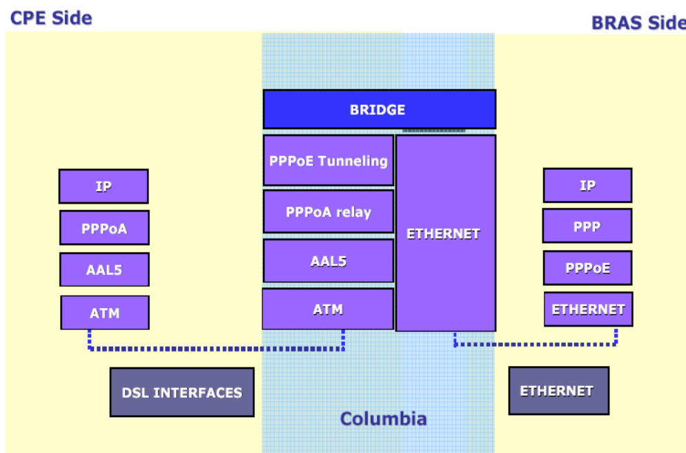
Рисунок 4-16: Стек протоколов для PPPoA to PPPoE Internetworking
