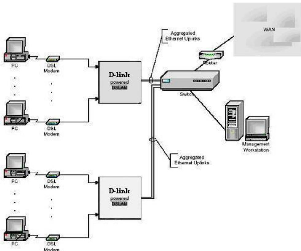
Рисунок 6-3: Использование Link Aggregation.
