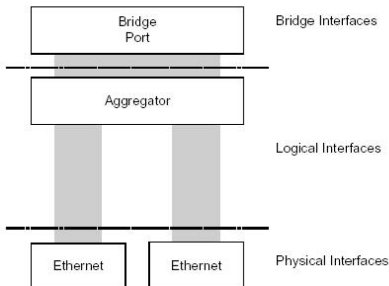
Рисунок 6-4: Стек интерфейсов DAS-3248 при использовании Link Aggregation.
