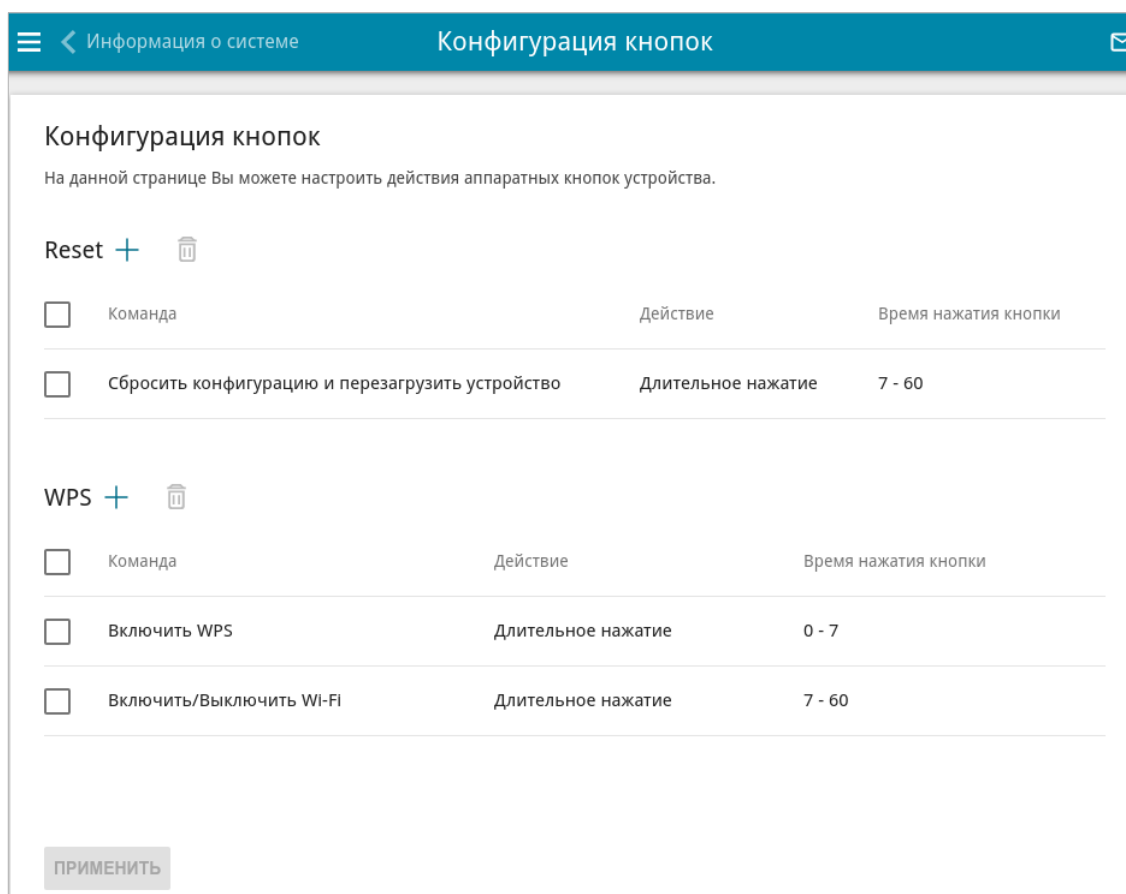
Рисунок 210. Страница Система / Конфигурация кнопок .
