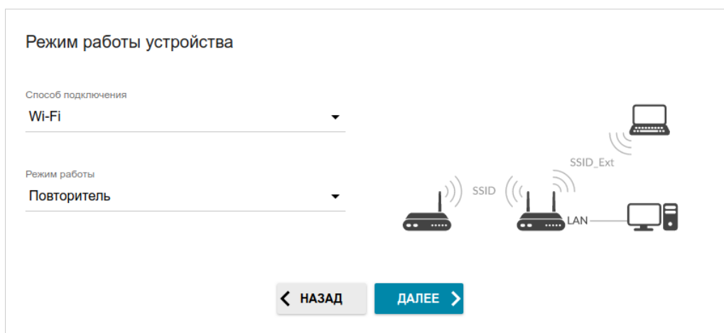
Рисунок 37. Выбор режима работы устройства. Режим Повторитель .
