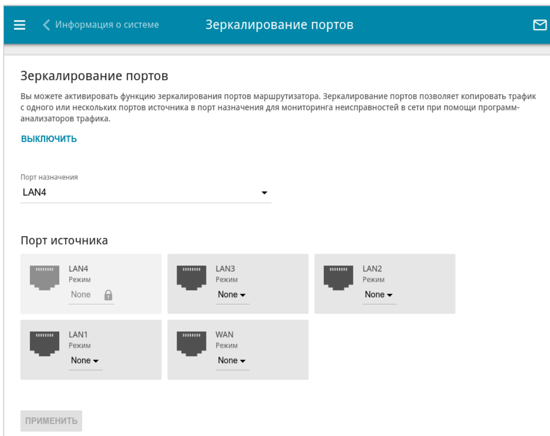
Рисунок 183. Страница Дополнительно / Зеркалирование портов .
