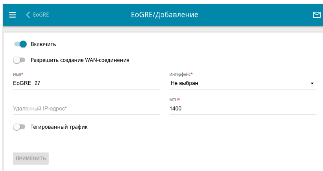
Рисунок 129. Страница добавления EoGRE-туннеля.
