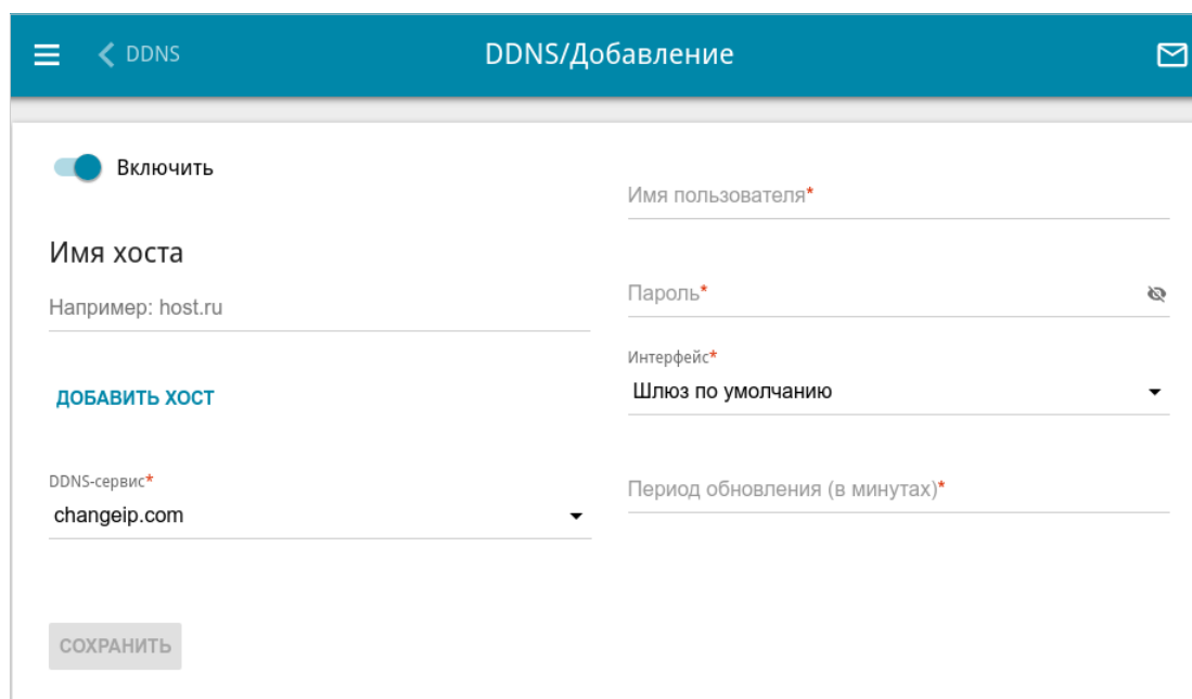
Рисунок 173. Страница добавления нового DDNS-сервиса.
