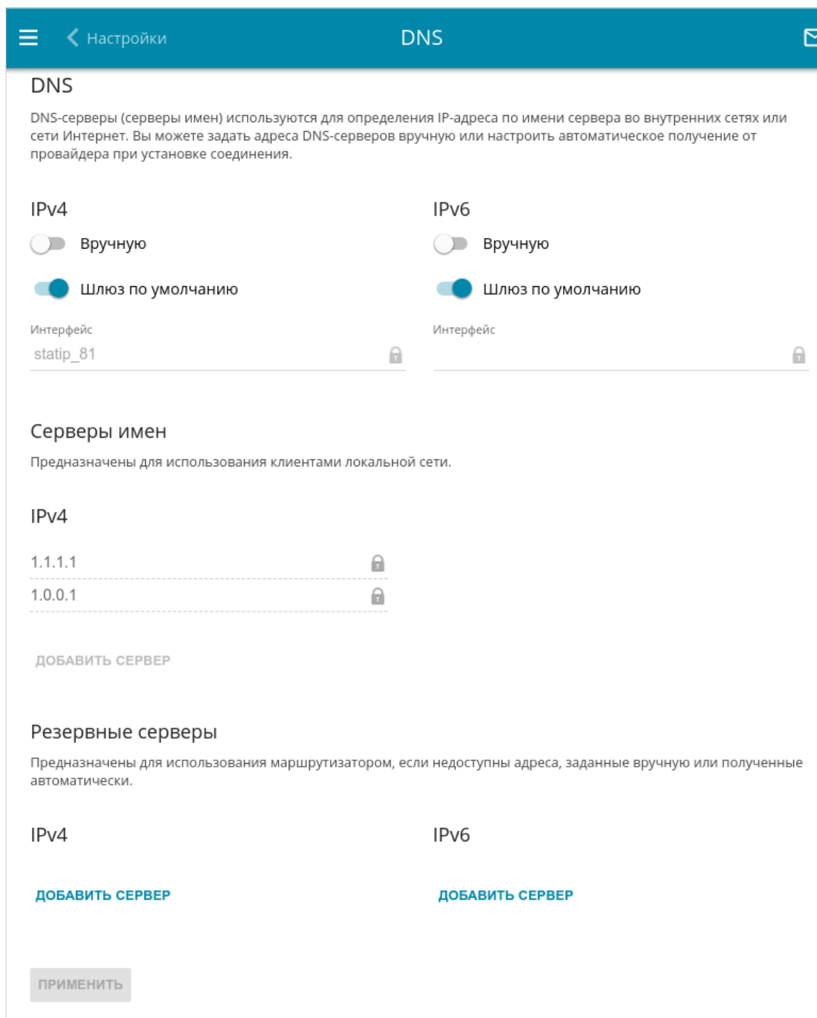
Рисунок 171. Страница Дополнительно / DNS .
