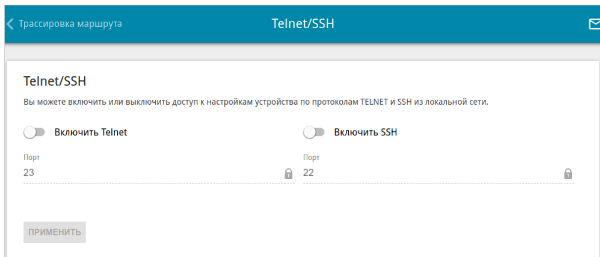
Рисунок 218. Страница Система / Telnet/SSH .
