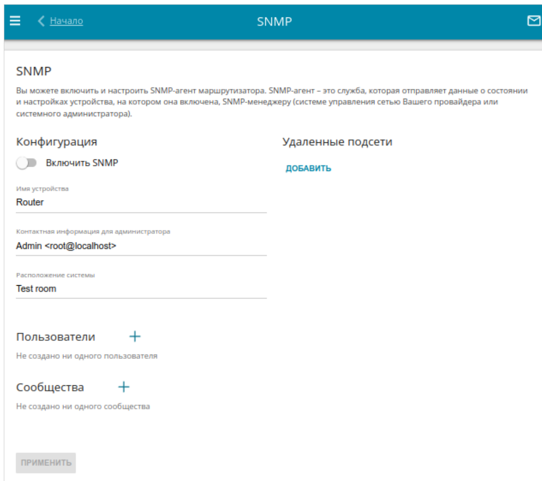
Рисунок 169. Страница Дополнительно / SNMP .
