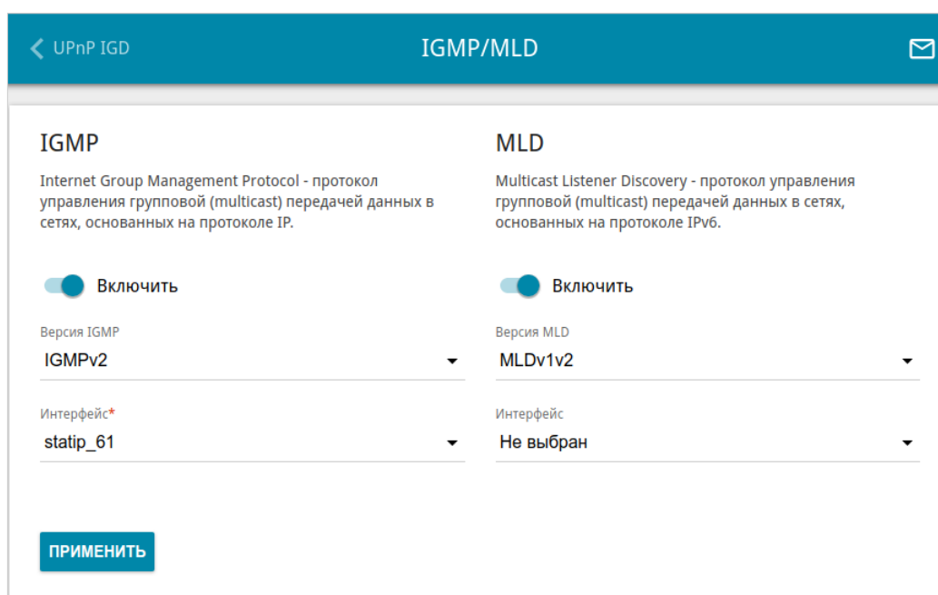
Рисунок 184. Страница Дополнительно / IGMP/MLD .
