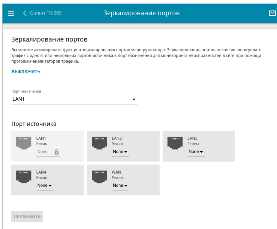
Рисунок 180. Страница Дополнительно / Зеркалирование портов .
