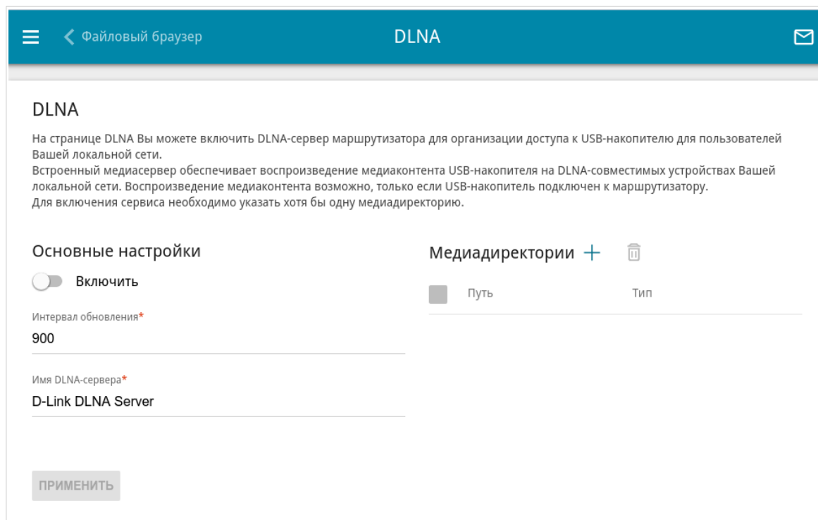
Рисунок 152. Страница USB-накопитель / DLNA .
