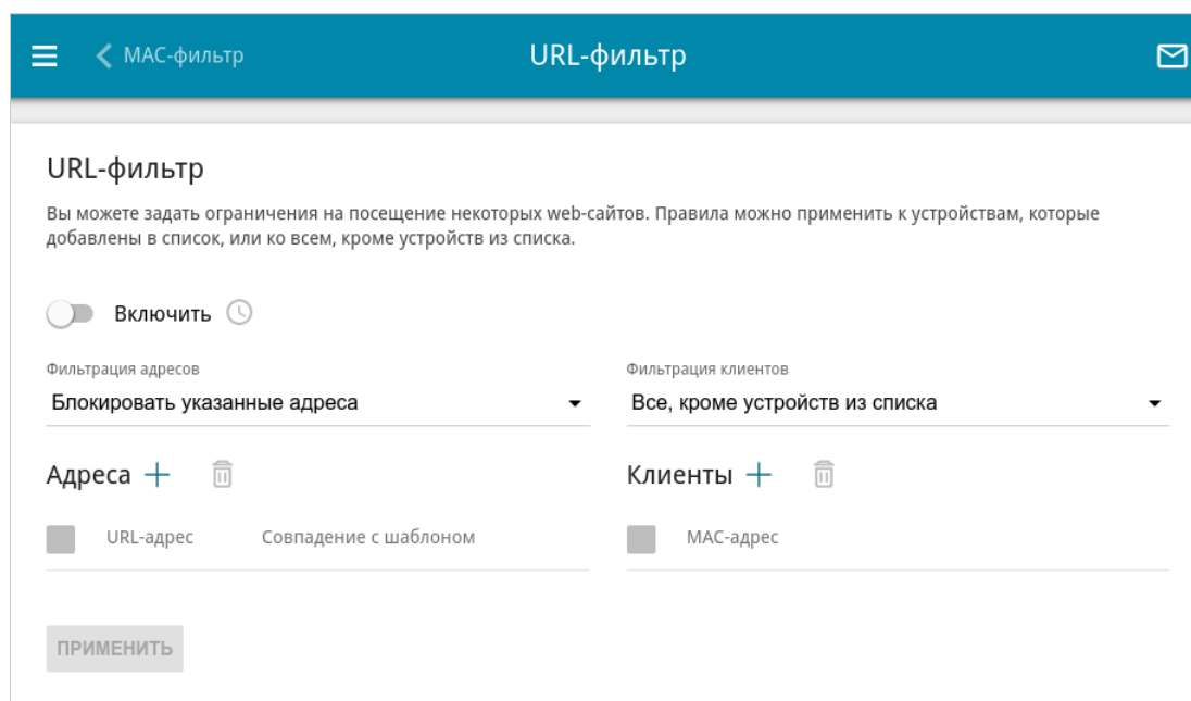
Рисунок 200. Страница Межсетевой экран / URL-фильтр .
