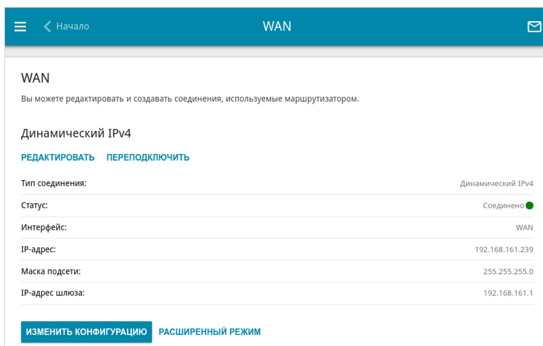
Рисунок 67. Страница Настройка соединений / WAN . Упрощенный режим.
