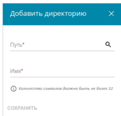
Рисунок 131. Добавление директории.
