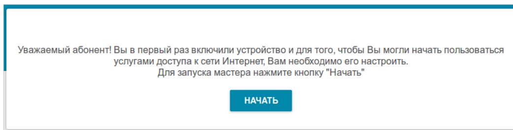
Рисунок 21. Запуск Мастера.
