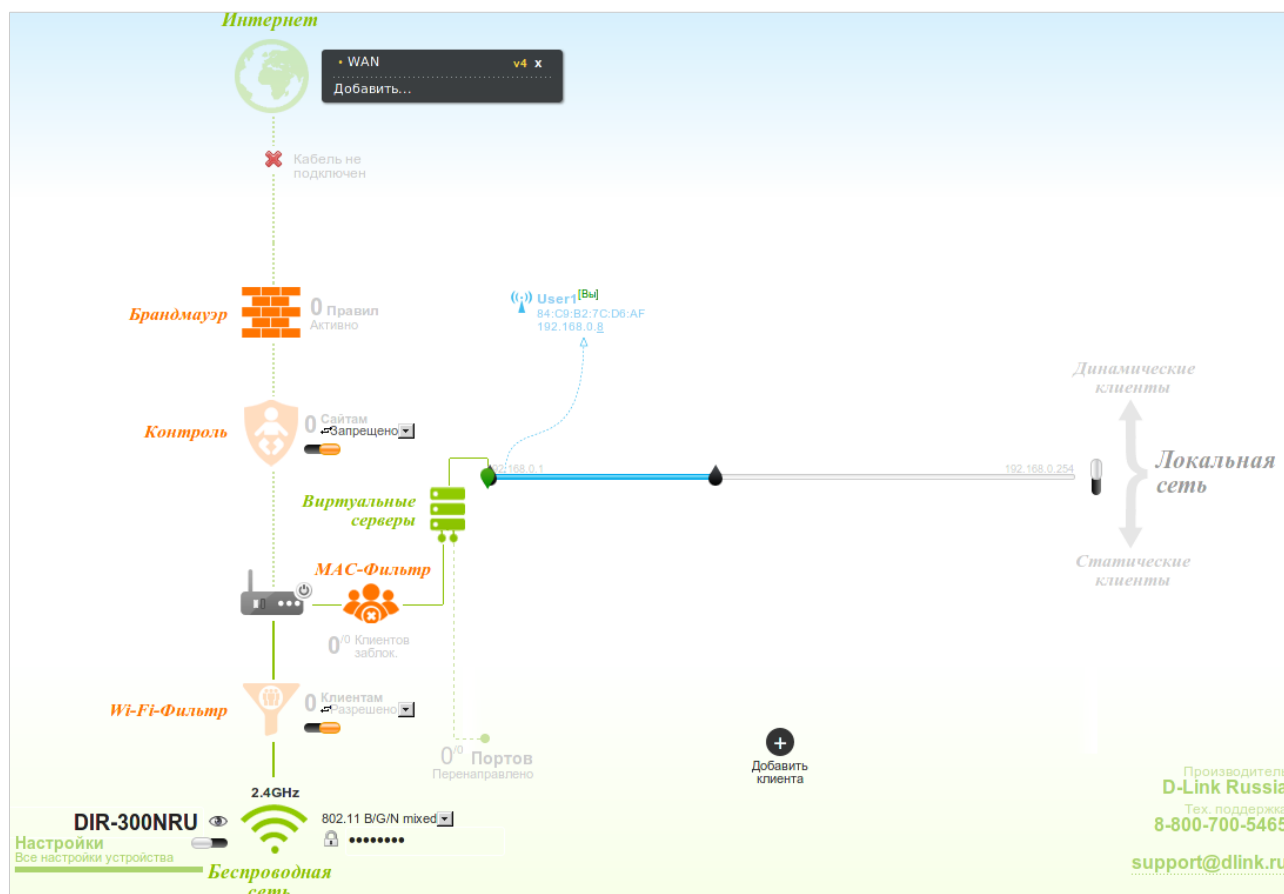
Рисунок 22. Страница Мониторинг .
