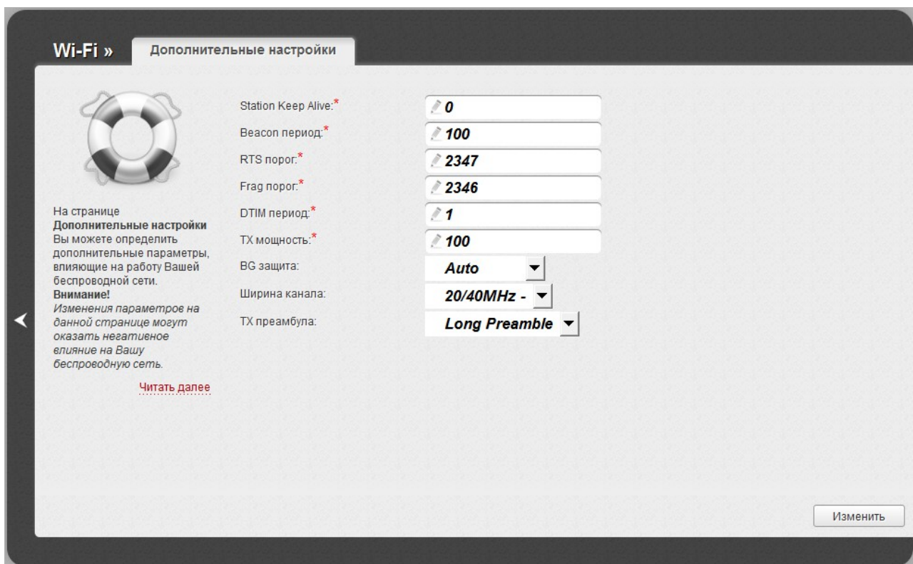
Рисунок 103. Страница дополнительных настроек для беспроводной сети.
