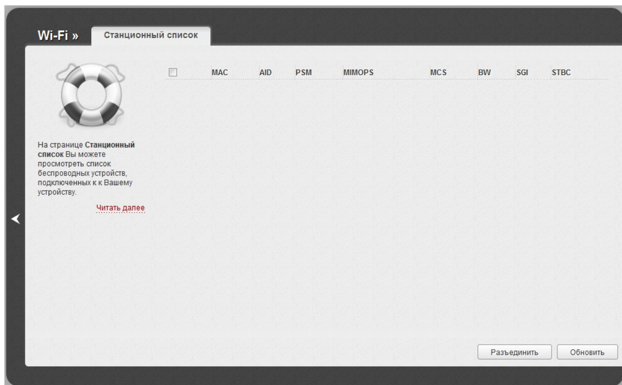
Рисунок 101. Страница для управления подключенными беспроводными устройствами.
