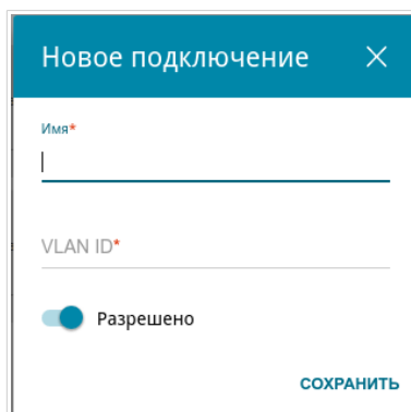
Рисунок 44. Добавление подключения.
