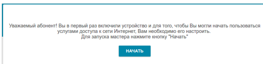
Рисунок 21. Запуск Мастера.
