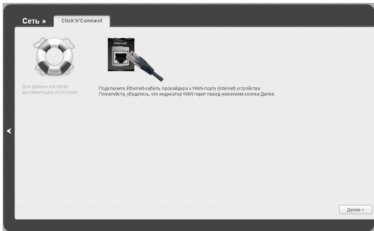
Рисунок 24. Настройка WAN-соединения.
