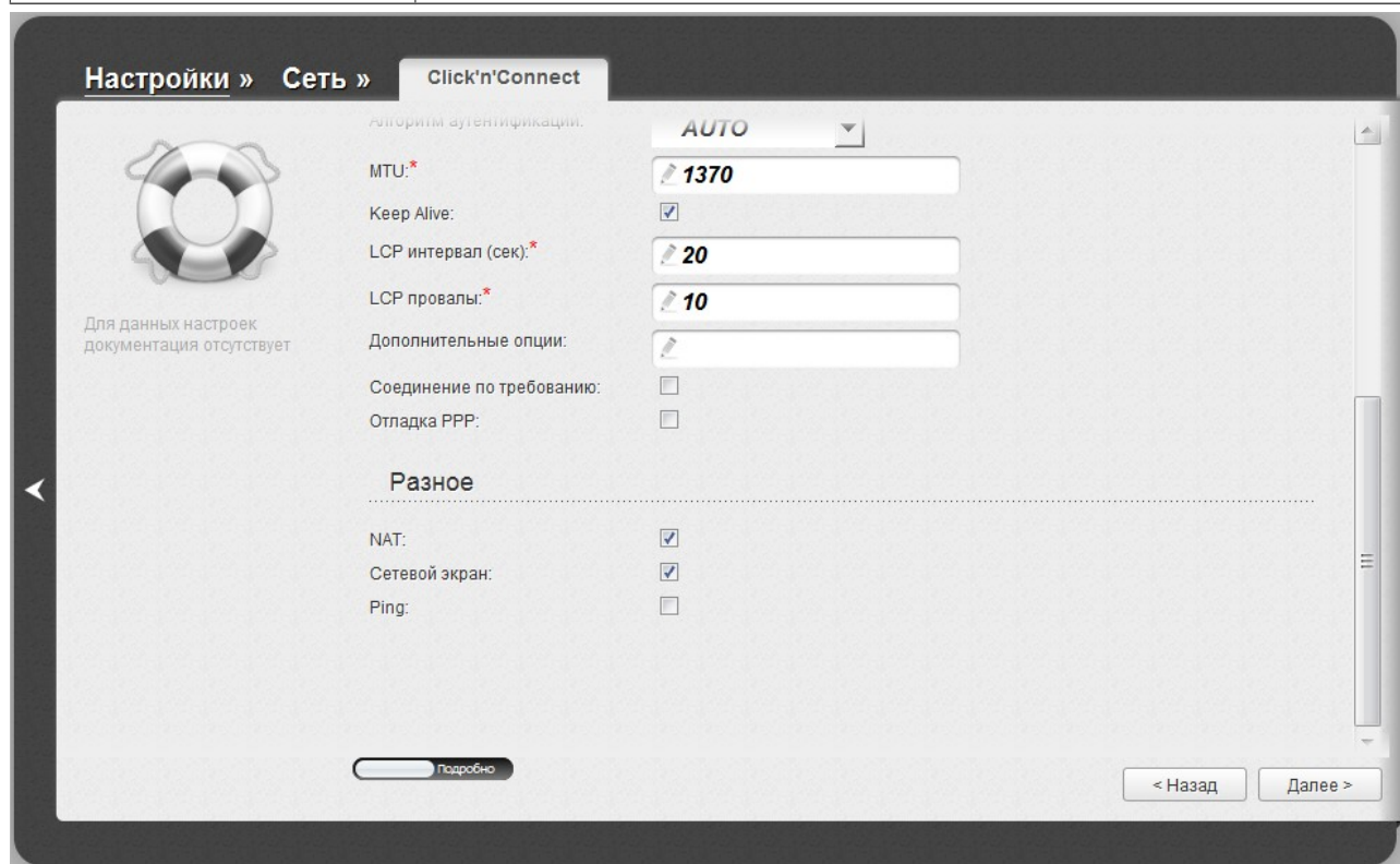
Рисунок 53. Настройка WAN-соединения типа 3G. Экспертный режим настроек. Раздел Разное .
