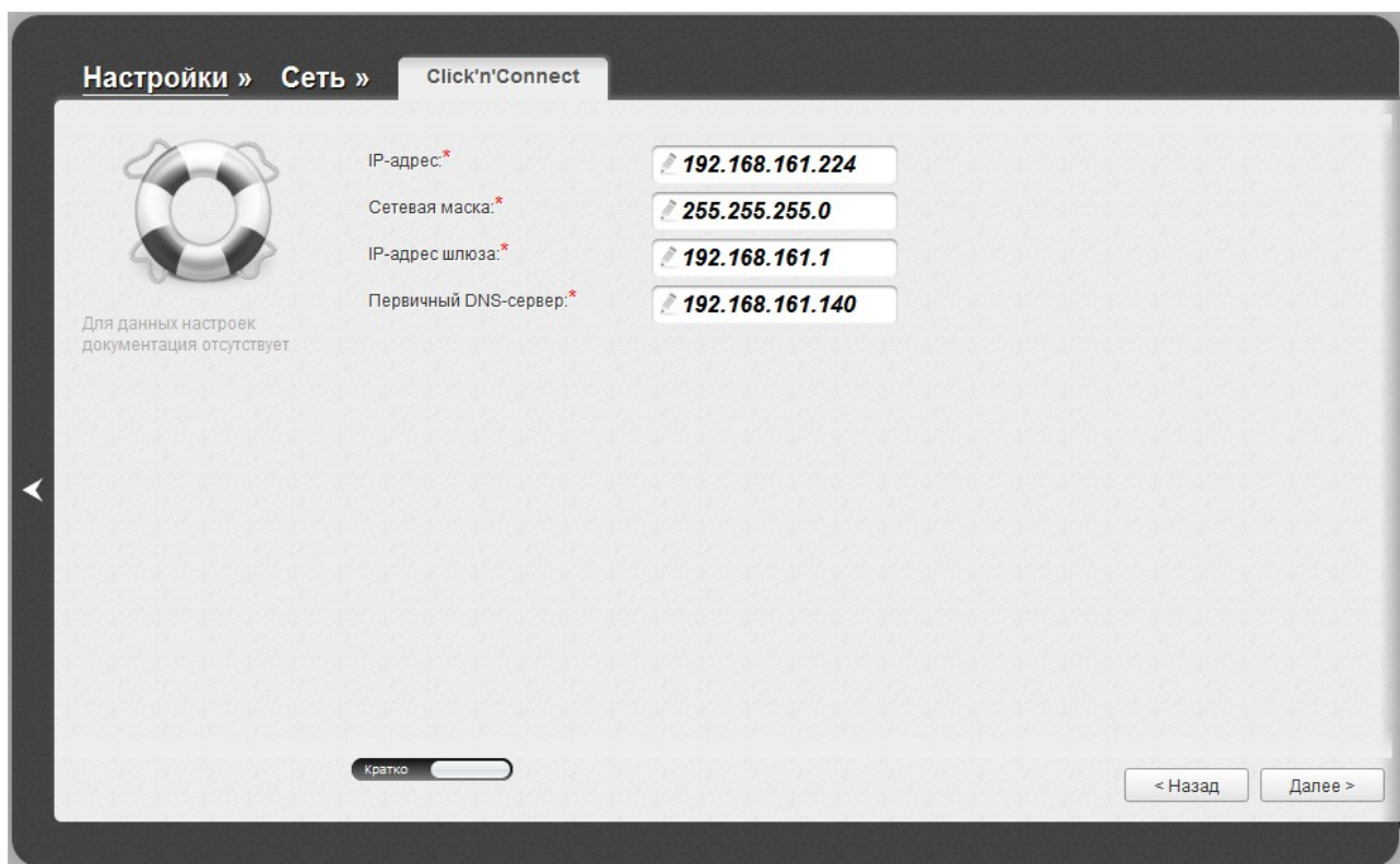
Рисунок 38. Настройка WAN-соединения типа PPTP + Статический IP.
