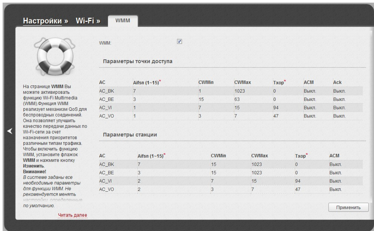
Рисунок 106. Страница для настройки функции WMM.
