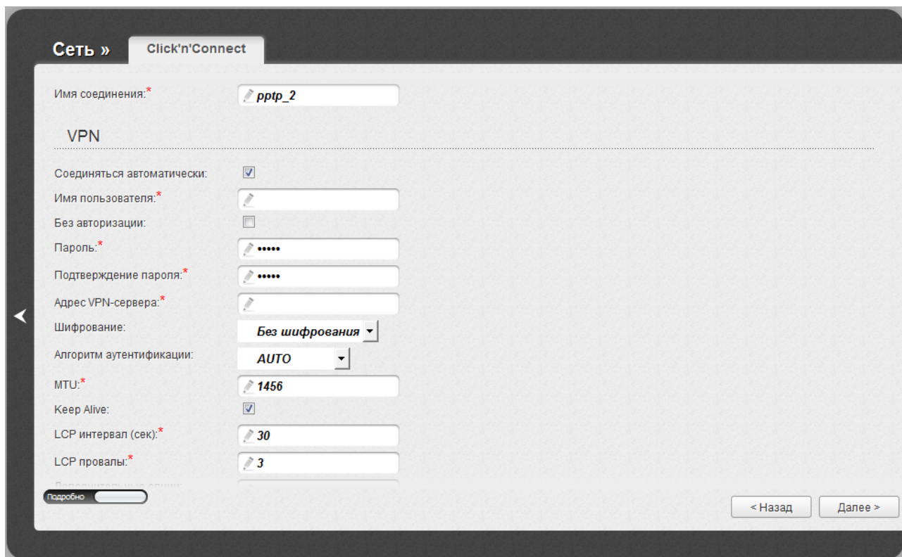
Рисунок 40. Настройка WAN-соединения типа PPTP. Экспертный режим настроек. Раздел VPN.
