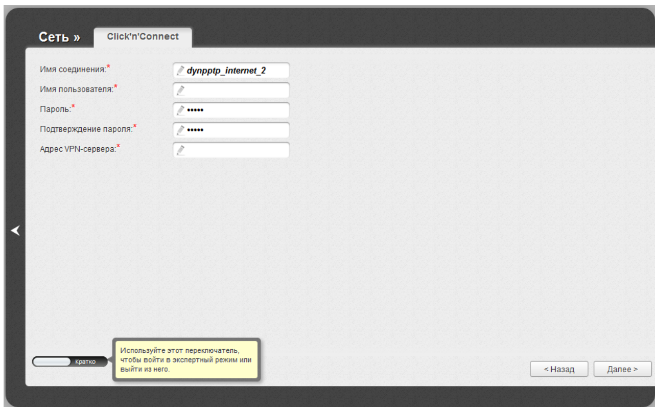
Рисунок 54. Настройка WAN-соединения типа PPTP + Динамический IP.
