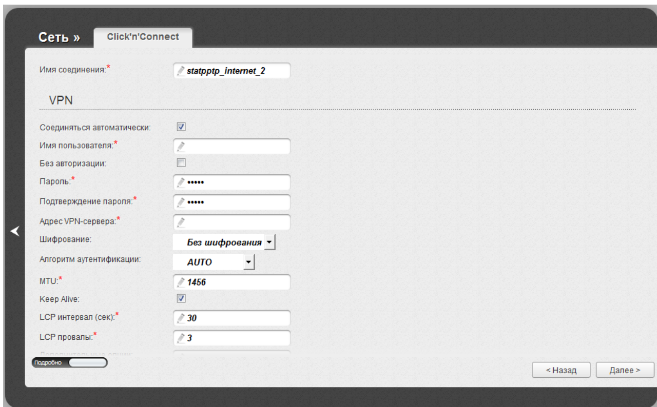
Рисунок 48. Настройка WAN-соединения типа PPTP + Статический IP. Экспертный режим настроек. Раздел VPN.
