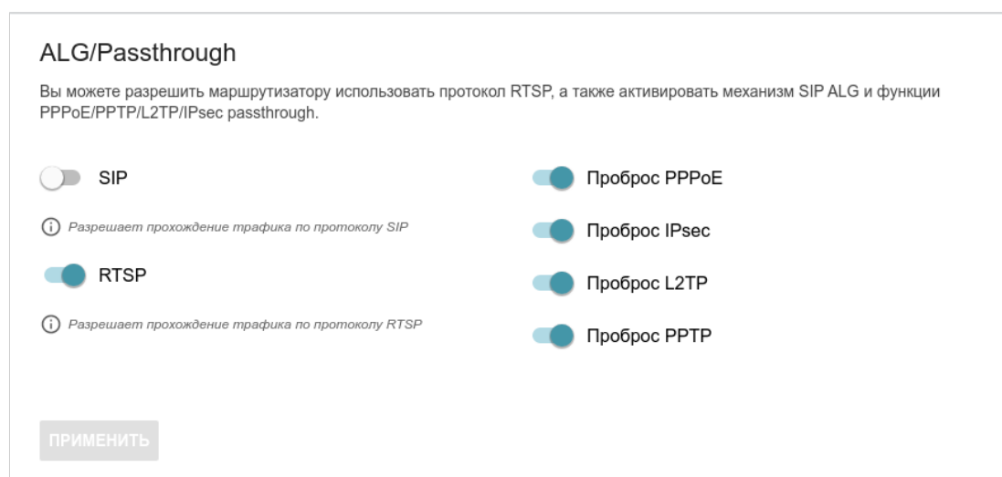
Рисунок 137. Страница Функции / Дополнительно / ALG/Passthrough .
