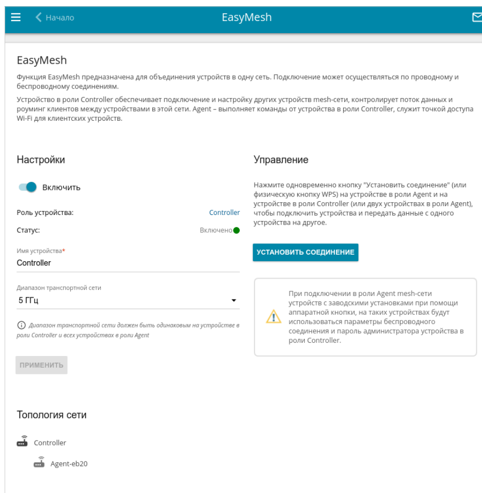
Рисунок 115. Страница Wi-Fi / EasyMesh .
