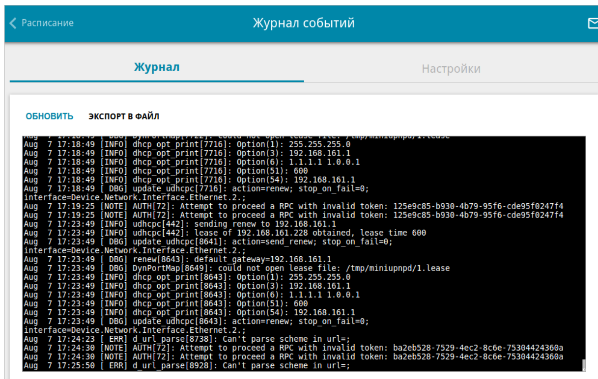
Рисунок 157. Страница Система / Журнал событий. Вкладка Журнал.
