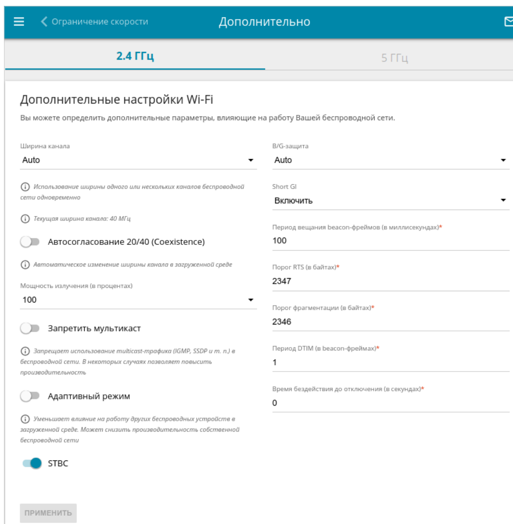
Рисунок 112. Страница дополнительных настроек для беспроводной сети.
