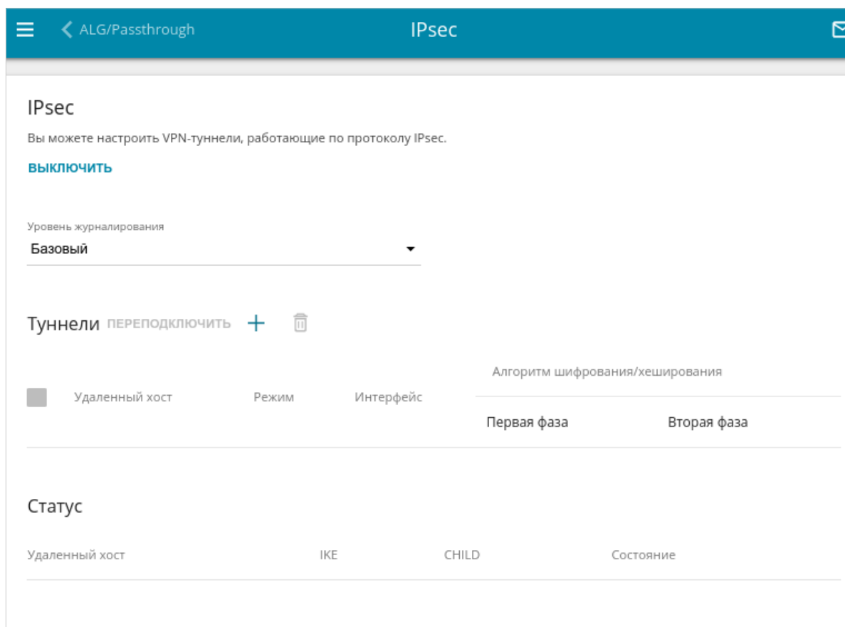
Рисунок 131. Страница Дополнительно / IPsec .
