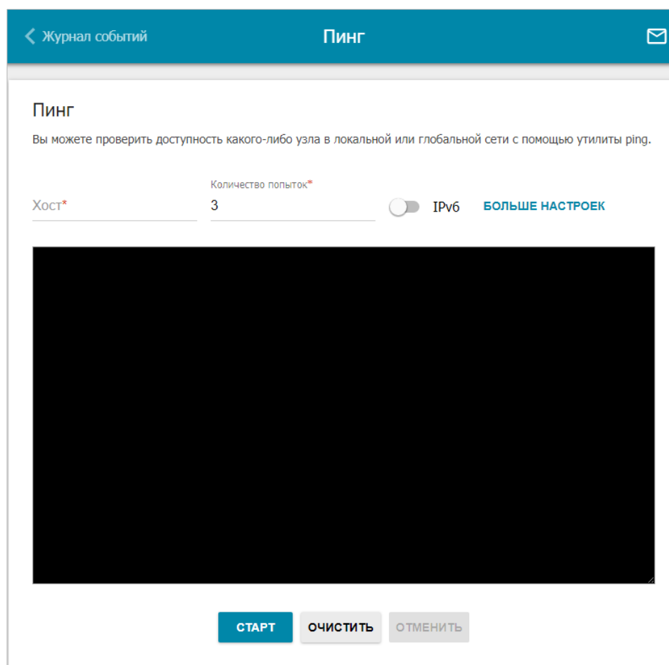
Рисунок 158. Страница Система / Пинг .
