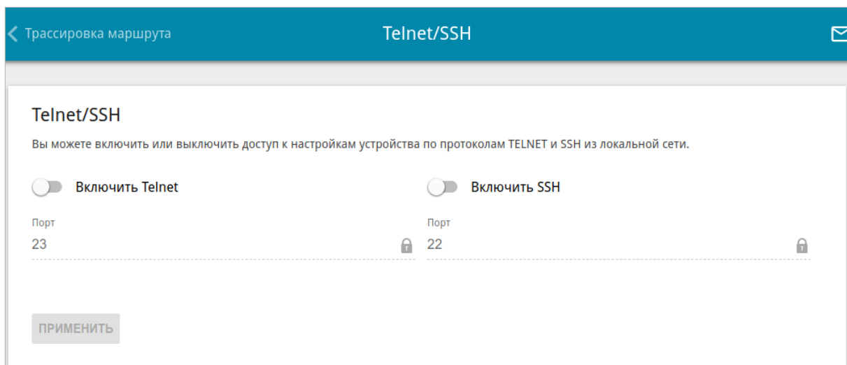
Рисунок 162. Страница Система / Telnet/SSH .
