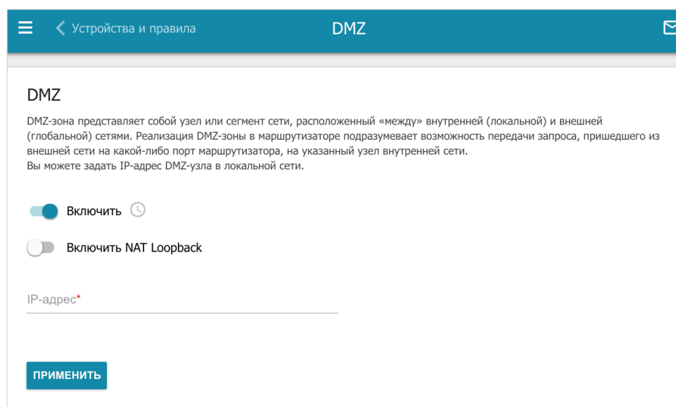
Рисунок 144. Страница Межсетевой экран / DMZ .
