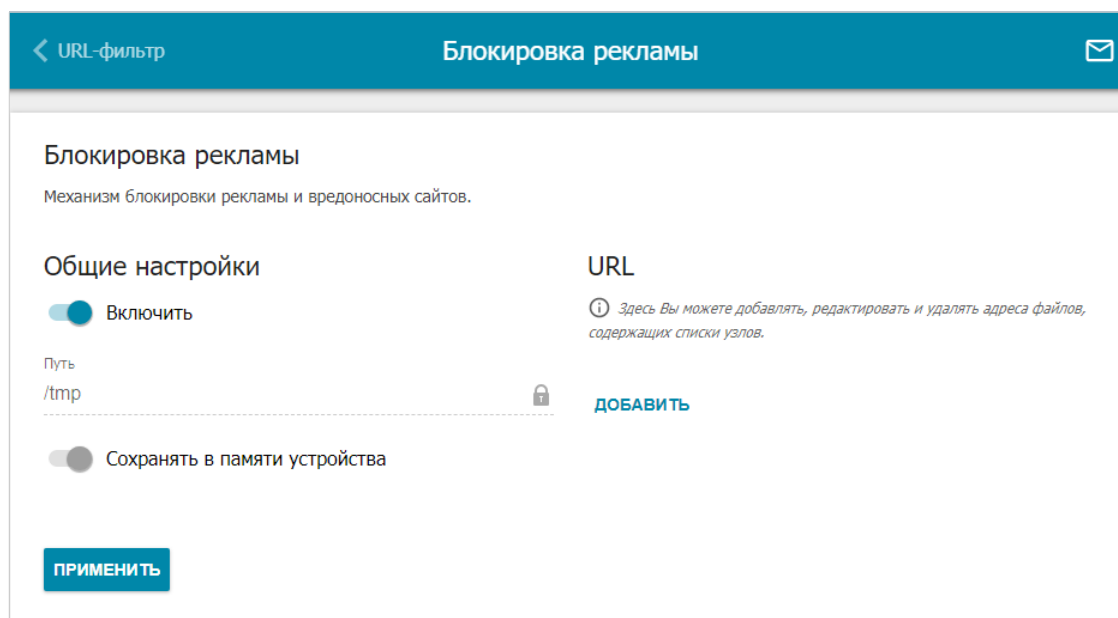
Рисунок 148. Страница Межсетевой экран / Блокировка рекламы .
