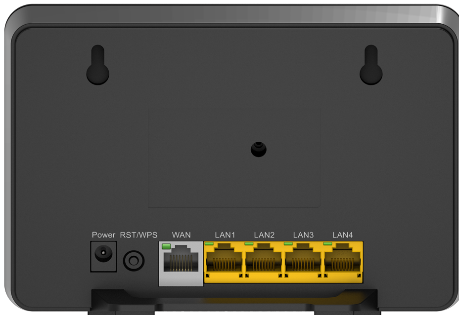
Рисунок 2. Вид задней панели.
