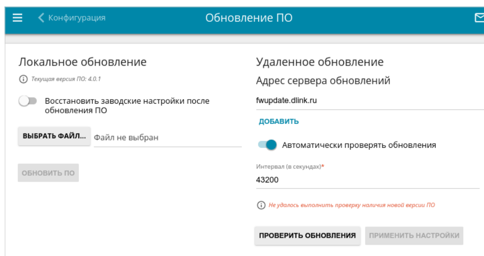
Рисунок 152. Страница Система / Обновление ПО .
