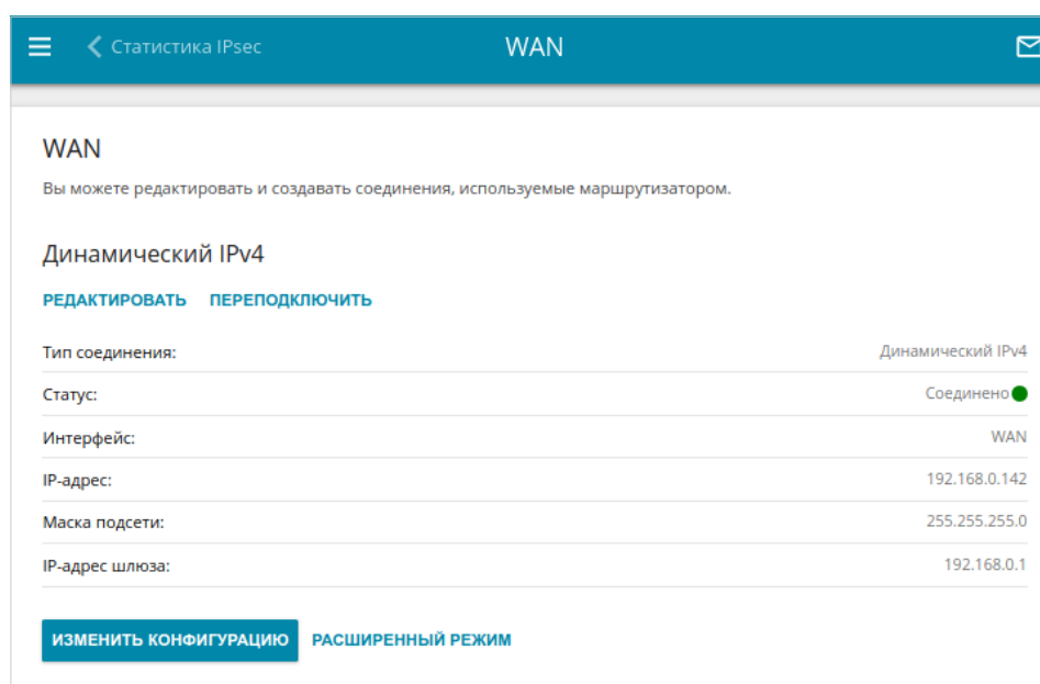
Рисунок 66. Страница Настройка соединений / WAN . Упрощенный режим.
