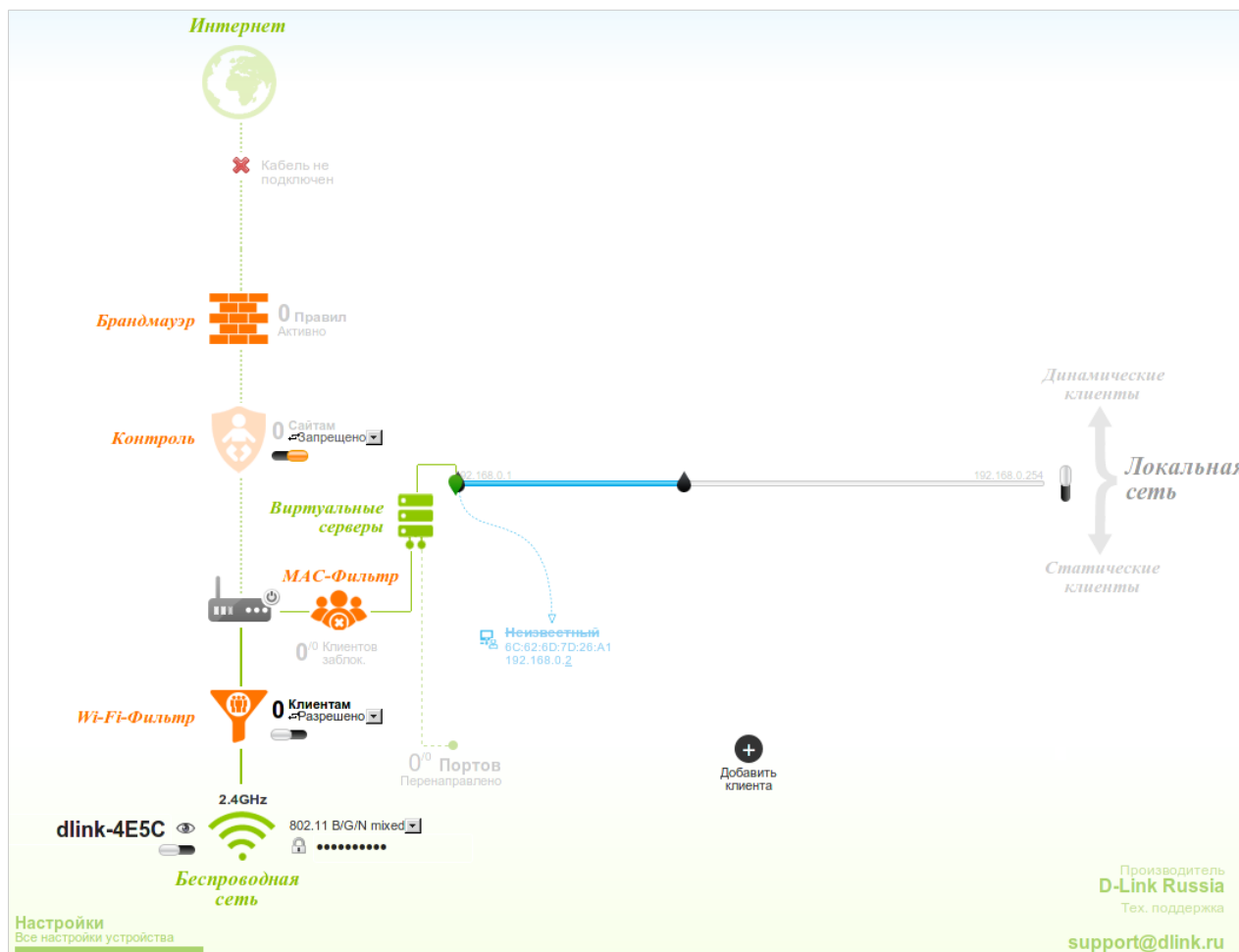
Рисунок 22. Страница Мониторинг .
