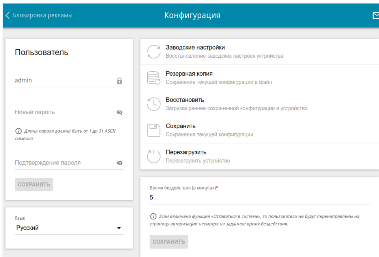
Рисунок 209. Страница Система / Конфигурация .
