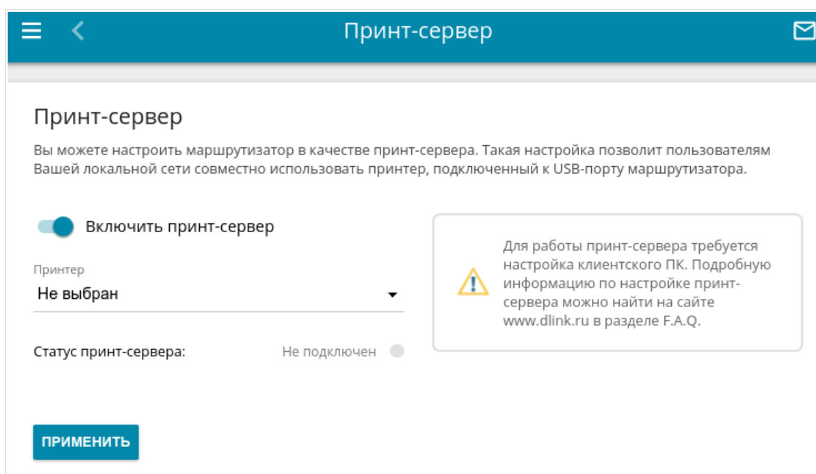
Рисунок 137. Страница Принт-сервер .
