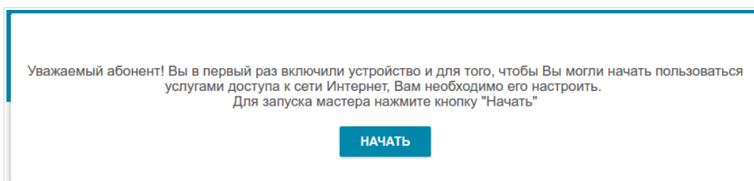
Рисунок 31. Запуск Мастера.
