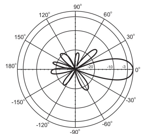
Направленность антенны в горизонтальной плоскости
