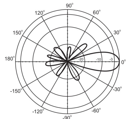
Направленность антенны в вертикальной плоскости
