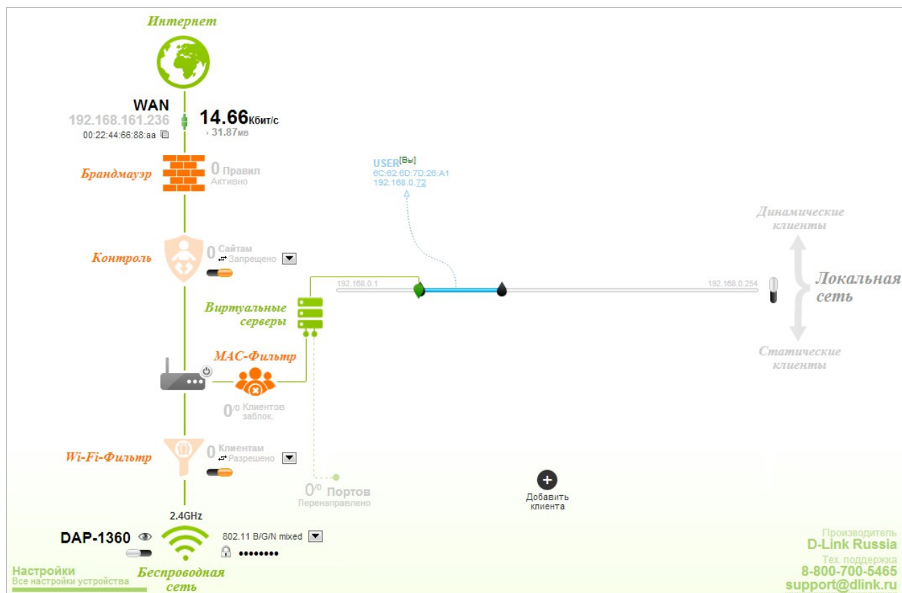
Рисунок 65. Страница Мониторинг .
