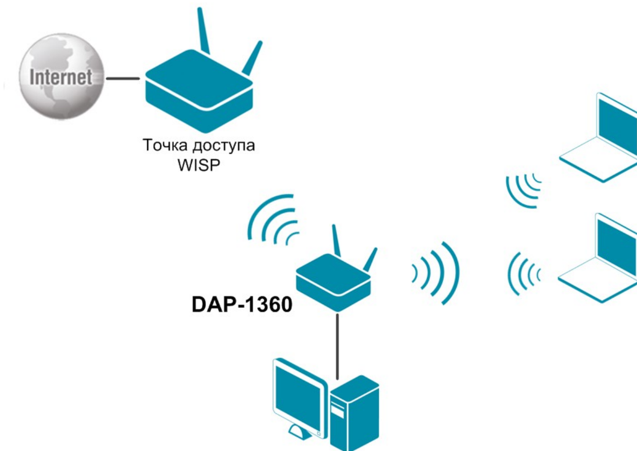
Рисунок 181. Подключение DAF-1360 в режиме маршрутизатора в качестве клиента.
