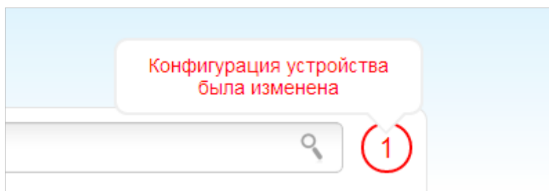
Рисунок 23. Уведомления web-интерфейса.
