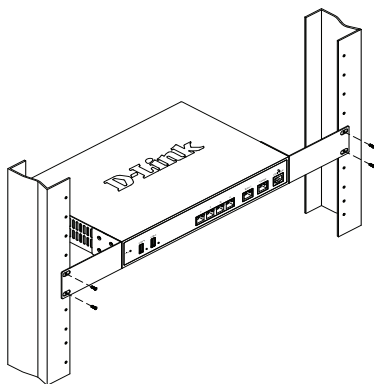
Figure 4. Installation du contrôleur sans fil dans un bâti de taille standard
