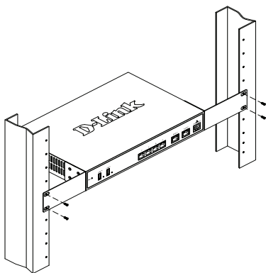
Figura 4. Instale el controlador inalámbrico en un estante de equipos de tamaño estándar
